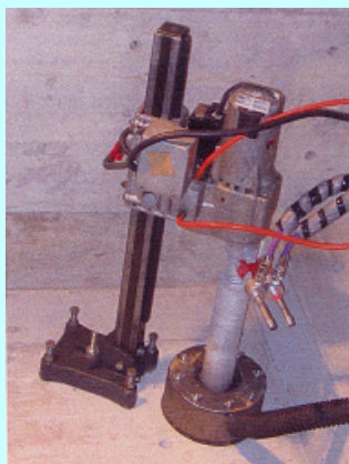
ダイヤモンドコアドリル
